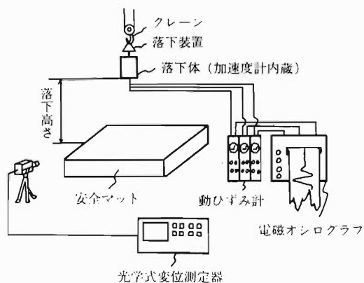
図3 実験概略図
