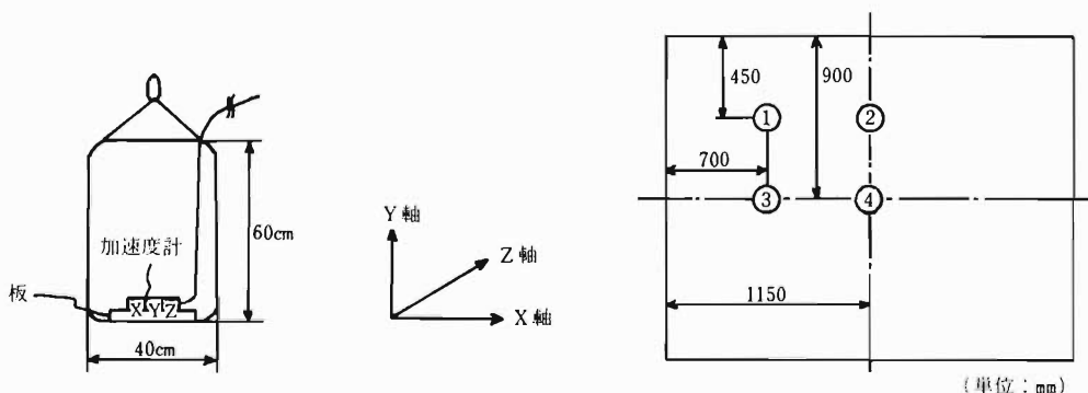
図2 落下体の構造
