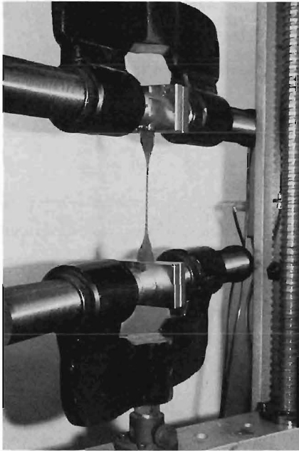
写真1 引張強さ等の測定状況
