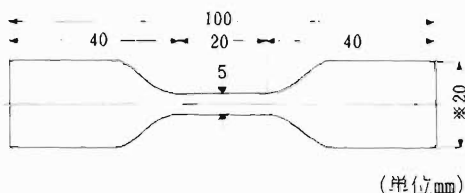
図1 ダンベル3号形の形状
