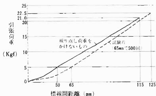
図3 繰り返し荷重試験結果(荷重曲線)
