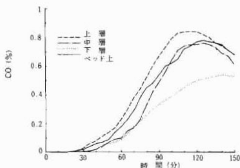
図4-5 CO濃度変化の比較
