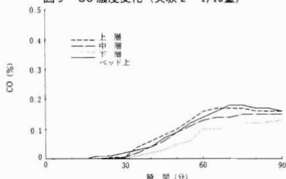
図10 CO濃度変化 (実験2 1/5量)
