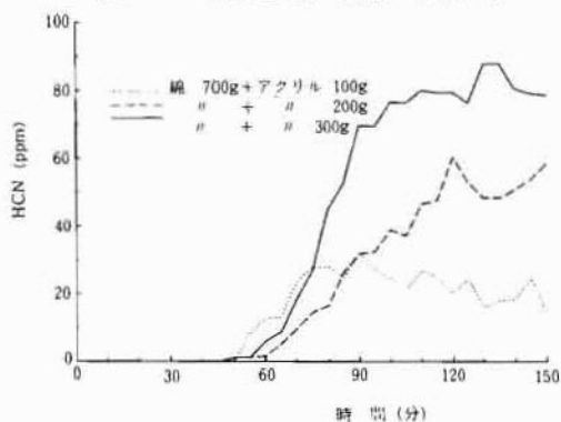
図12 HCN濃度変化の比較 (実験3)
