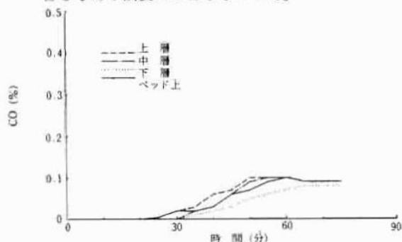
図9 CO濃度変化 (実験2 1/10量)
