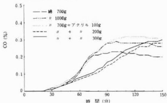
図11 CO濃度変化の比較 (実験3)
