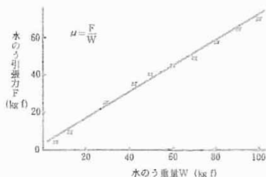
図3 水のう底面と接地面との摩擦係数測定結果
