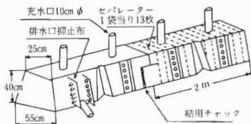
図1 漏油拡散防止水のうの構造 (2袋連結した状況)
