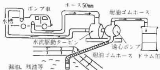
図6 油処理の構想図
