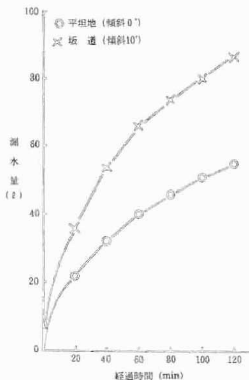
図2 水のうの布目からの漏水量 (一袋当り)
