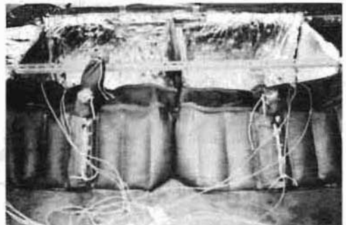
写真8 耐火性能実験のため熱電対取付けた状況
