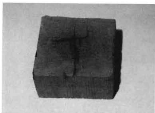
写真5 角材の内部の炭化状況(断面) (9cm角, 雰囲気170°C, 48時間加熱)
