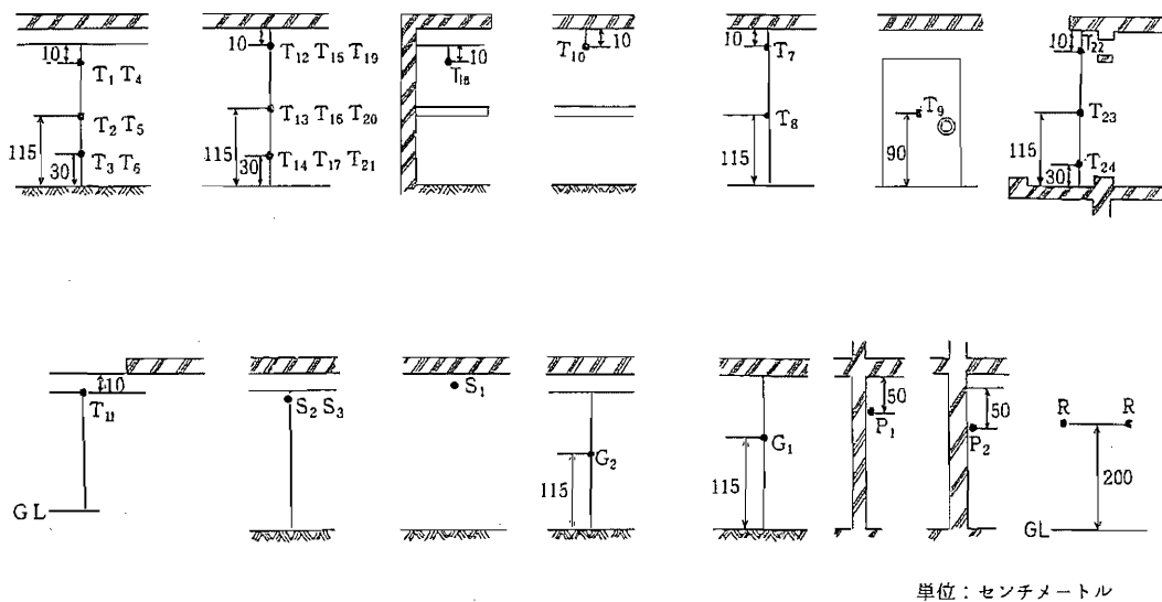
図4 測定点配置状況 (実験1 立体)
