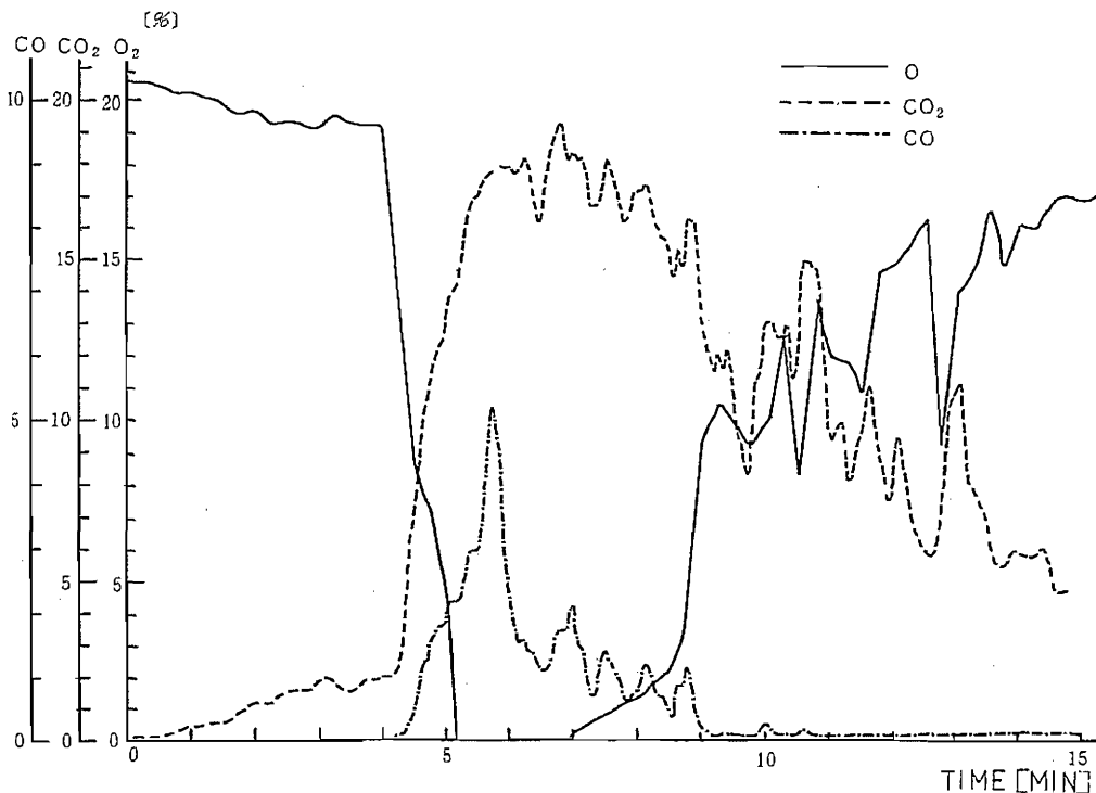
図13 ガス濃度測定結果(実験 1) 1階6畳間
