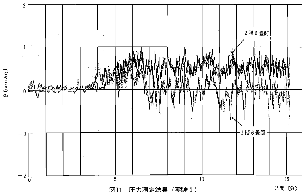
図11 圧力測定結果 (実験1)
