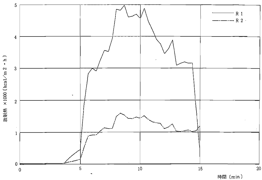
図15 放射熱測定結果 (実験 1)
