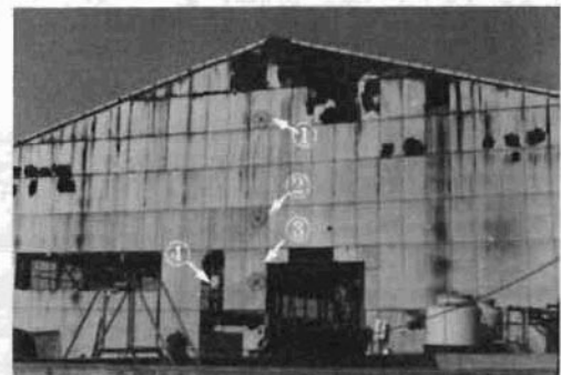
①②③……標的1.2.3.④放水衝撃力測定装置
