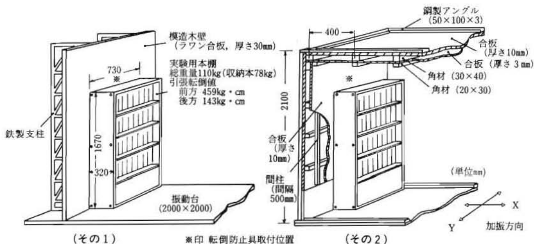
図1 振動実験セット
