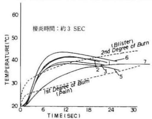
図5 残留熱試験
