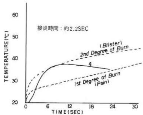
図6 残留熱試験
