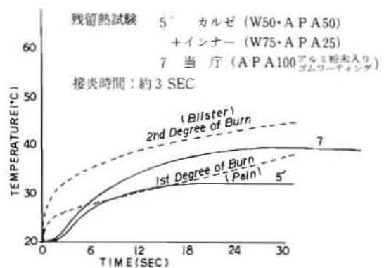
図7 残留熱試験
