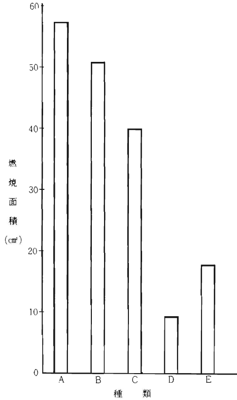
図9 燃焼試験
