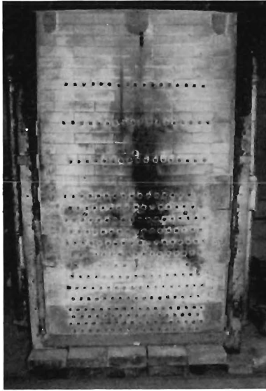
写真 1 防火力試験炉
