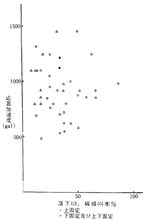
図15 D戸柵（木製）
