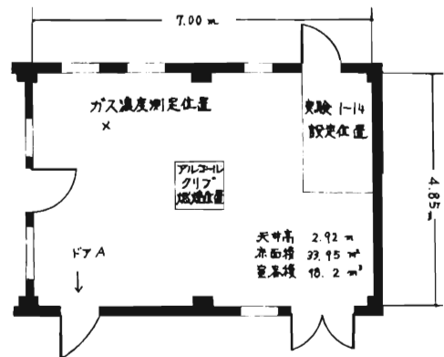
図1 火災室平面概要図
