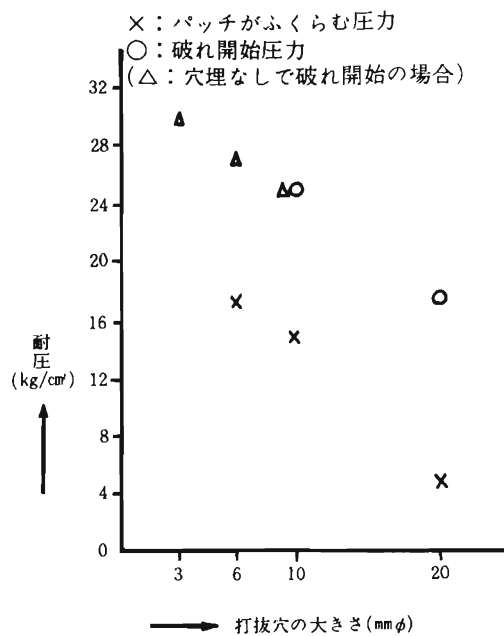
図10 ホースジャケット表面及び内張りゴムの両面にパッチを張った場合
