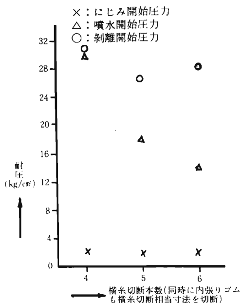
図8 互縫いでパッチ二重張りの耐圧
