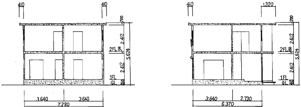
A-A 断面図
