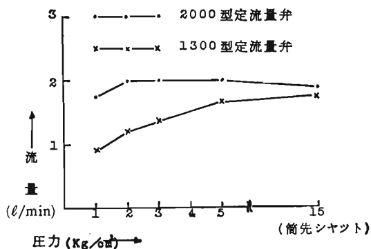
図-2 65mmホース
