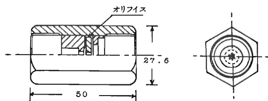
図-1 定流量弁
