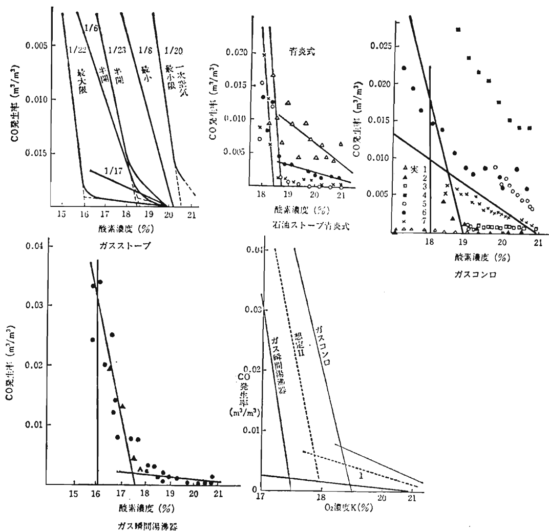
図 5 CO—O 2 特性
