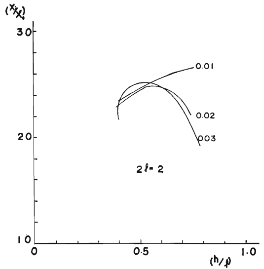
第10図 X_i/X_o \sim h/l 曲線 ( 2l=2 )
