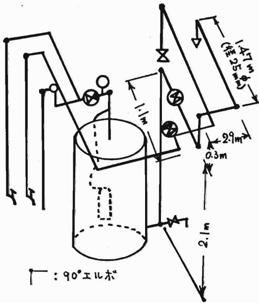
図4 配管図
