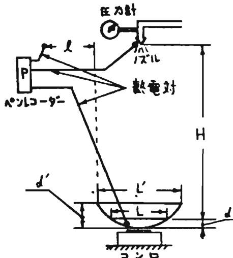
図 9 天ぷら油の消火実験
