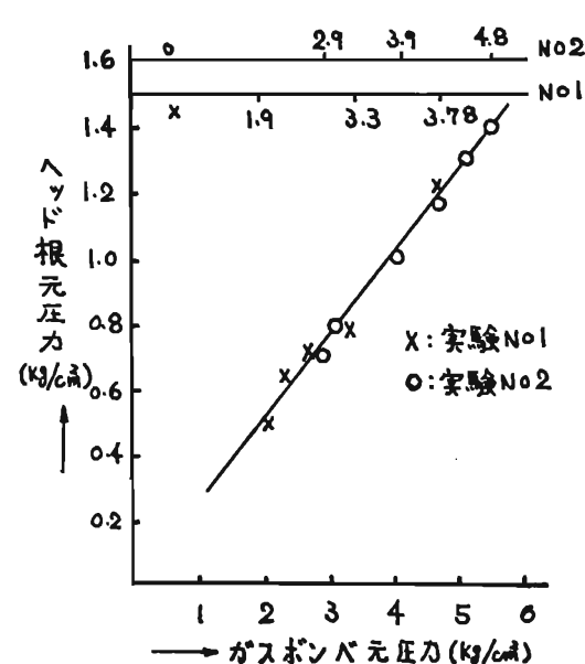
図 3 配管の損失圧力
