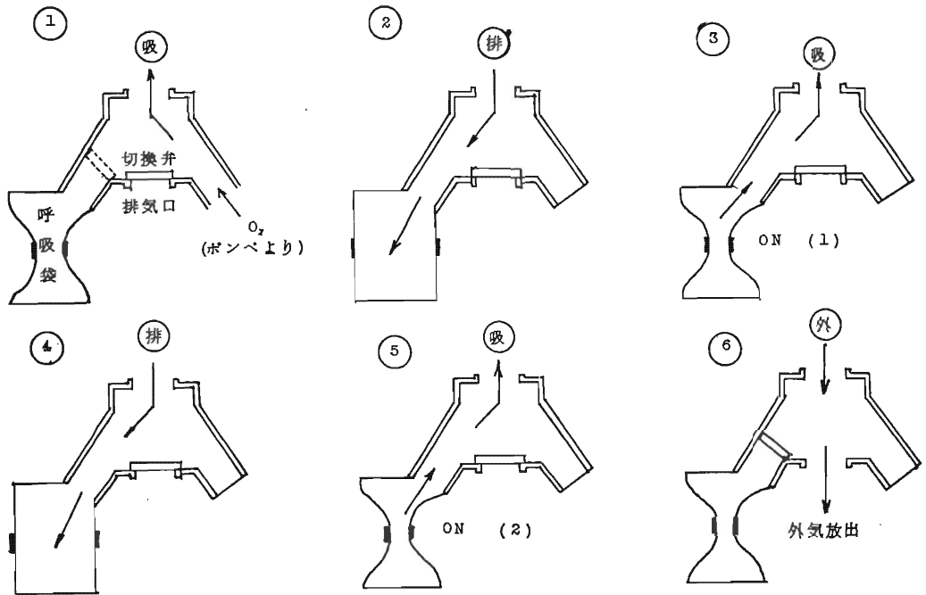
図2 切換弁作動状況
