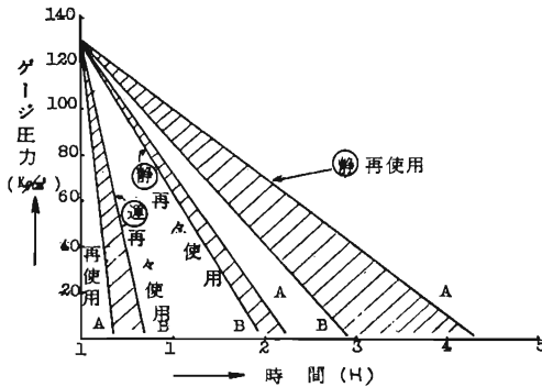
図一八 吸気量による使用可能時間
