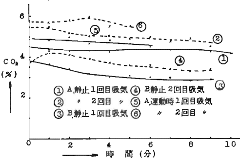
図-4 呼気再使用時における静止一運動時の C O 2 濃度
