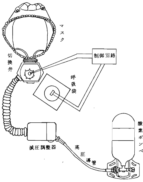
図-1 呼気再使用式酸素呼吸器の概要
