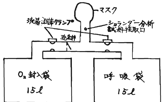
図2. 実験装置
