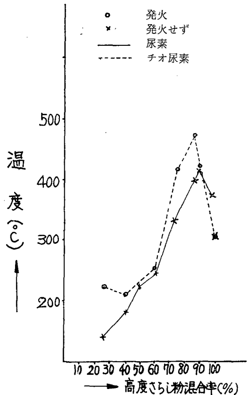
図2 高度さらし粉と尿素・チオ尿素との混触による跳熱性
