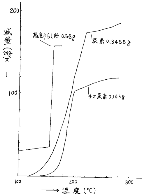
図3 熱天秤による加熱試験
