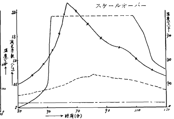
第8図 発煙物質の発煙特性と温度曲線
