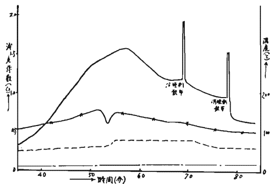
第22図 消煙剤による消煙効果と温度曲線
