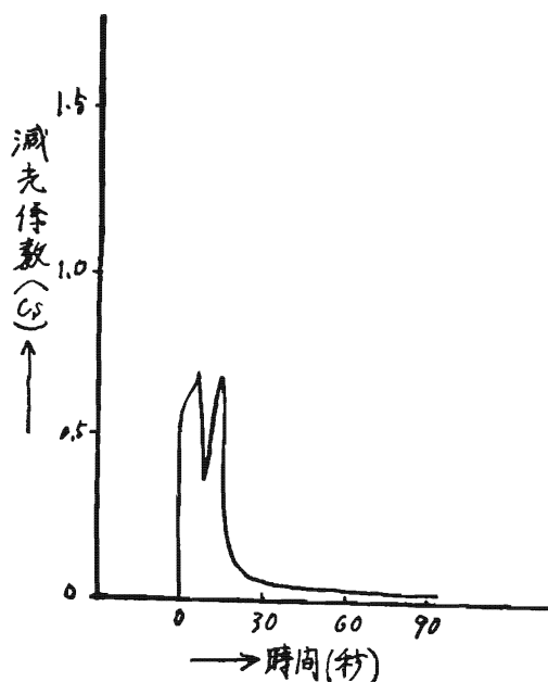
第14図 水噴霧の減光係数の変化 散布量 11.6\text{ l}
