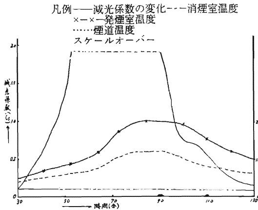
第5図 発煙物質の発煙特性と温度曲線
