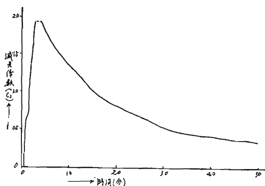
第15図 水噴霧による減光係数の変化 (エアロゾルを形成した場合)
