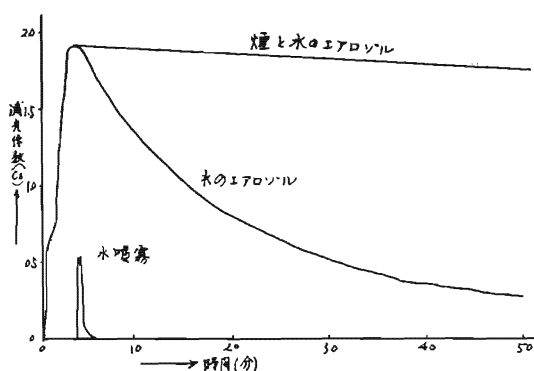
第16図 煙と水とのエアロゾルを形成した場合の C_s の変化
