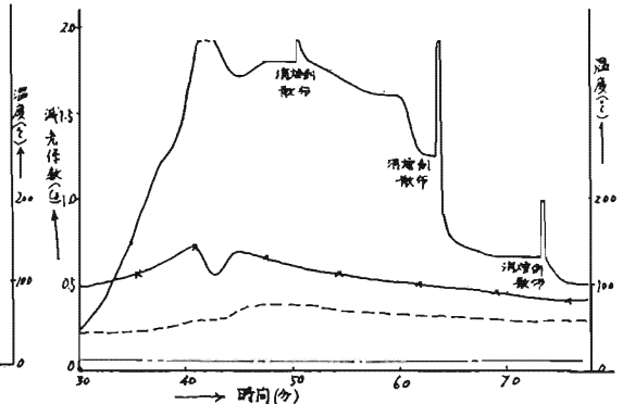
第24図 消煙剤による消煙効果と温度曲線
