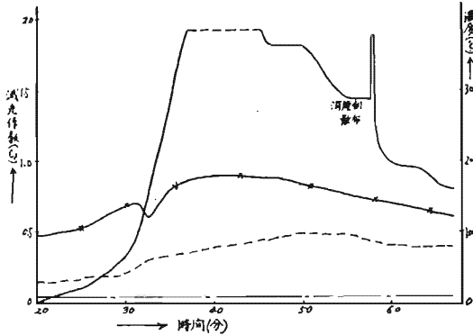
第28図 消煙剤による消煙効果と温度曲線
