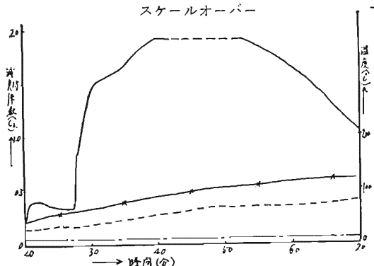
第13図 発煙物質の発煙特性と温度曲線
