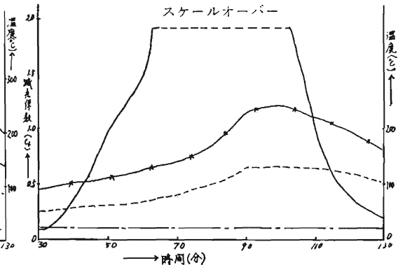
第9図 発煙物質の発煙特性と温度曲線
