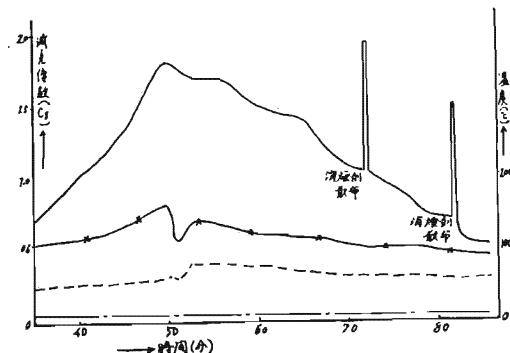
第19図 消煙剤による消煙効果と温度曲線
