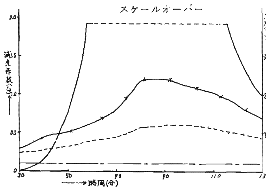
第6図 発煙物質の発煙特性と温度曲線
