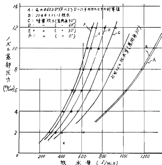
第2図 放水量曲線
