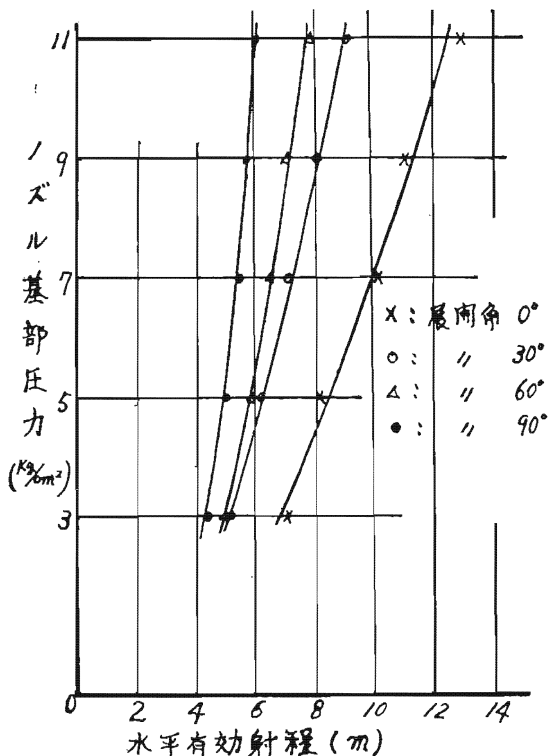
第3図 噴霧水平有効射程
