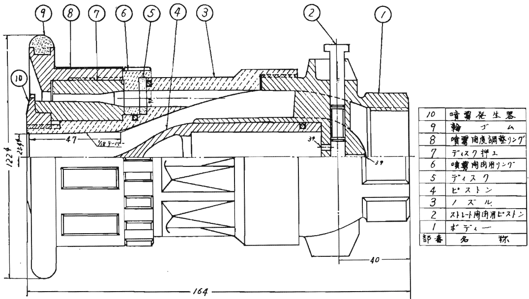
第1図 可変ノズル組立図
