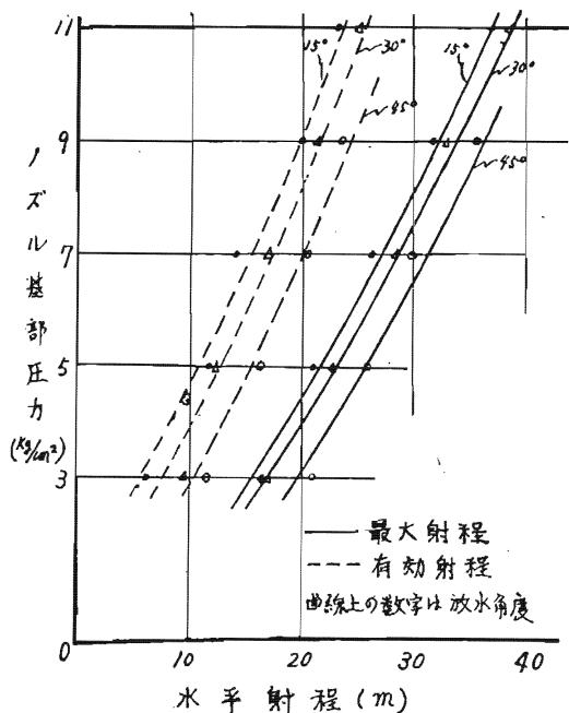
第7図 噴霧水平射程
