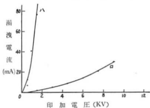
第20図 救助用ロープの耐電圧特性（50cm）
