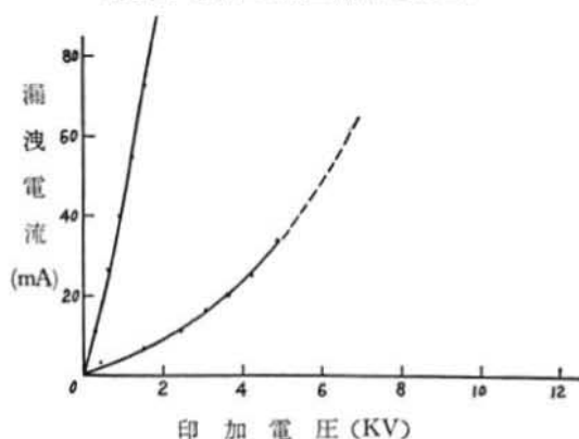
第26図 腰綱の耐電圧特性 (200cm)
