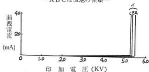
第5図 耐熱服 (地) の耐電圧特性
