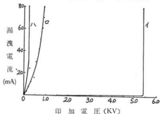
第5図 耐熱服 (地) の耐電圧特性
