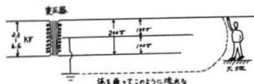
第30図 感電回路
