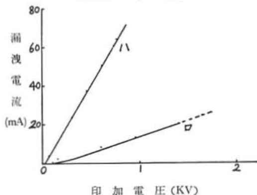
第9図 ネオプレン防火服(地)の耐電圧特性 —試料1cm×10cmの場合—
