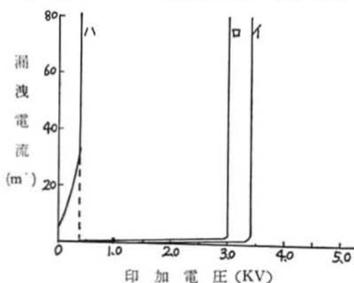
第3図 アルミックス防火服 (地) の耐電圧特性
