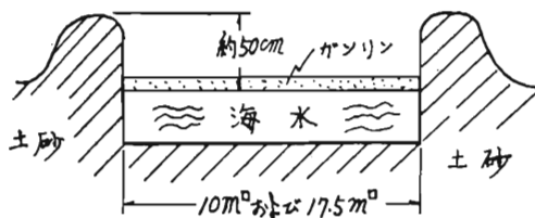
第2図 油面の造设法
