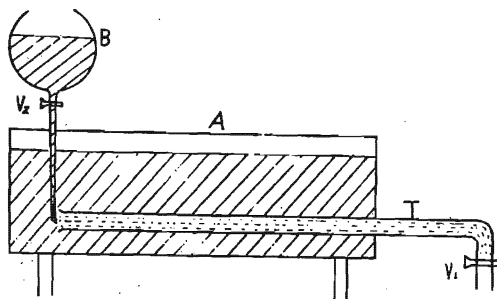
第1図 レイノルズ実験
