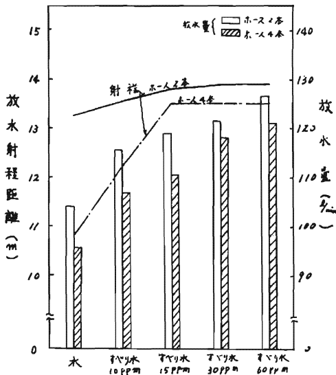
第7図 放水量、放水射程距離の測定
