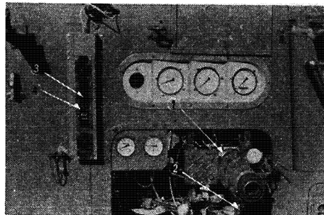
写真1 流量計の取付状況
