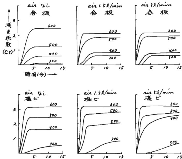
第5図 煙濃度
