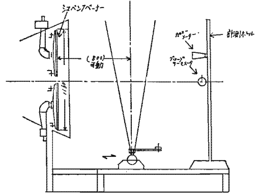
第1図 実験概要図
