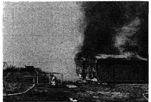
写真2 実験状況 (水噴霧発生装置1.2列放水の状態)
