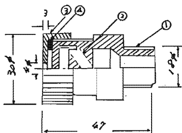
第8図 噴霧ノズル
