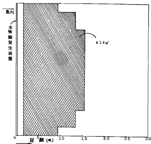
第9-5図 (ノズル圧力 3\text{kg}/\text{cm}^2 風速 7.5\text{m}/\text{sec} )
