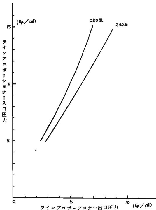
図2-3 ラインプロポーションナー圧力損失 (技術資料より)
