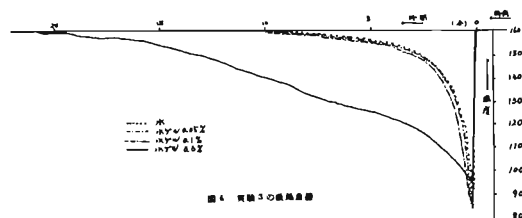
図4 実験3の吸熱曲線
