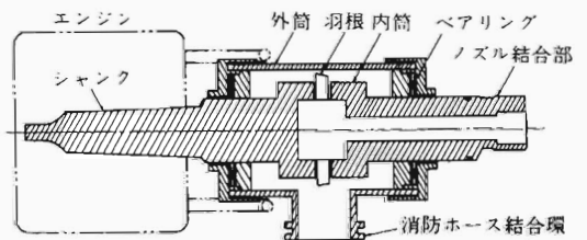
図1 回転軸部送水管
