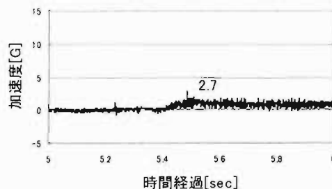
図11 副ノズルで放水時の衝撃加速度
