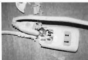
写真19 実験6の状況
