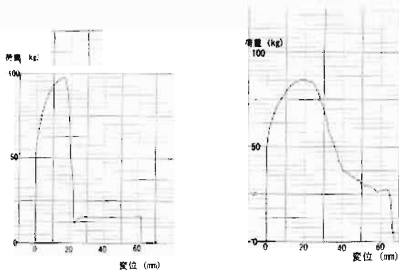
図2 変位-荷重曲線(試験体1)
