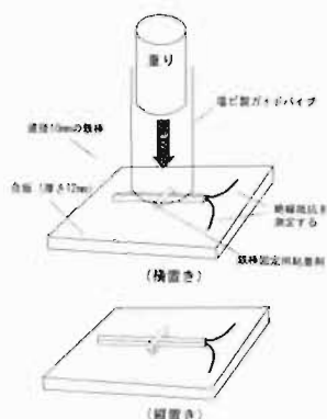
図1 落下実験の設定
