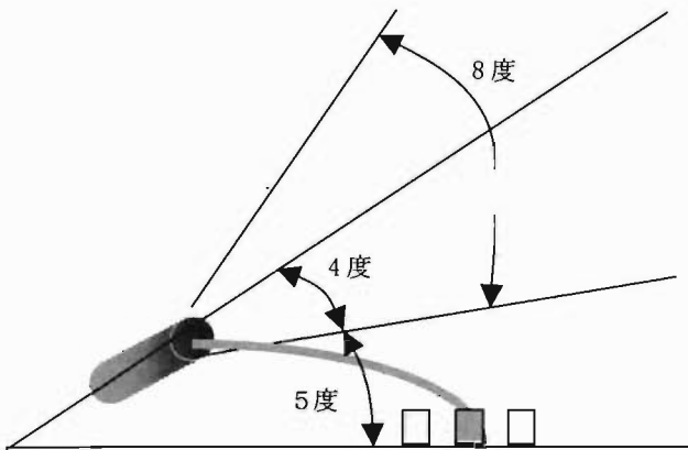
図7 横から見た放水展開角
