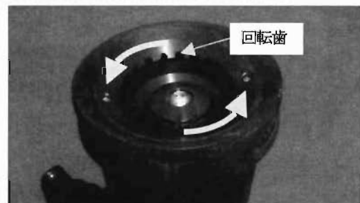
写真4 ターボジェットノズル 放水口
