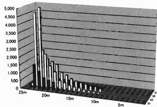
図 2-2 実験 3-2 の散水分布 (放水形状：ストレート)
