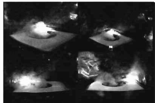
写真3 A社製簡易消火具で一方向から放射した場合1回目（消火開始2秒後）
