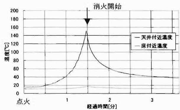
図3 実験1 (消火距離 1m) A社製簡易消火具で一方向から放射した場合2回目の温度変化
