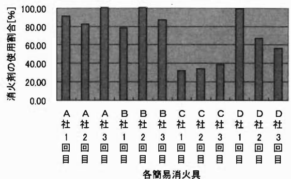
図 13 くずかごの火災を移動しながら放射した消火剤使用割合 (消火距離 1m) (くずかごの火災)
