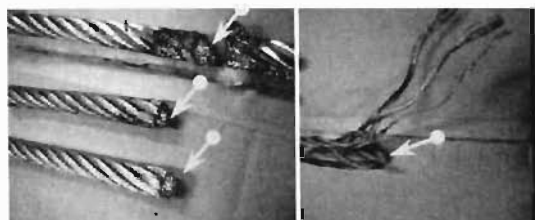
写真20 ワイヤー切断状況
