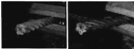
写真26 ワイヤ切断面 (左：エンジンカッター、右：プラズマ金属加工機)
