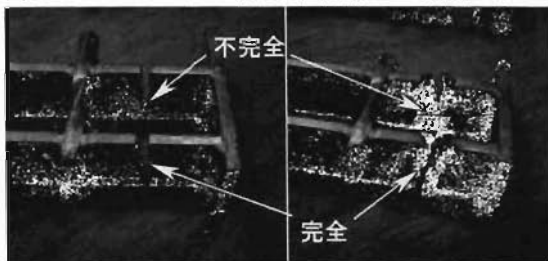
写真28 切断不完全な状況(左：ディスクグラインダー、右：プラズマ金属加工機)
