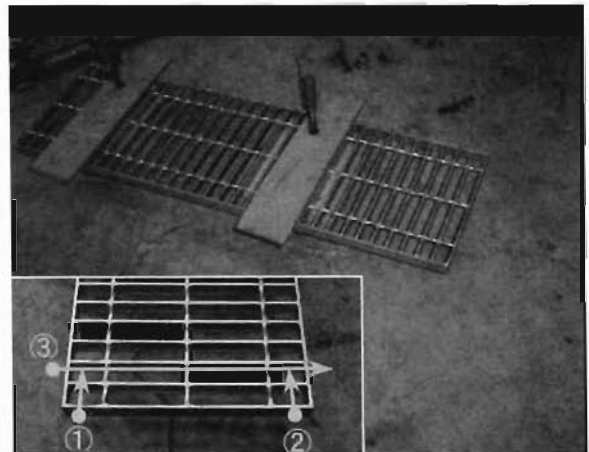
写真15 ワイヤー (矢印: 切断位置、方向 番号: 順番)
