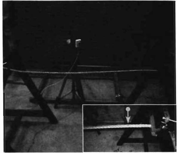
写真13 ワイヤー (矢印: 切断位置、方向)
