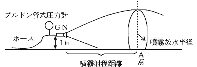
図3 噴霧射程距離
