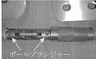
写真14 ボールプランジャー式ストッパー機構
