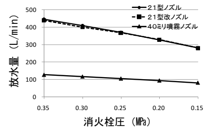
図6 呼称65 3本延長
