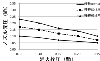
図29 21型改ノズル
