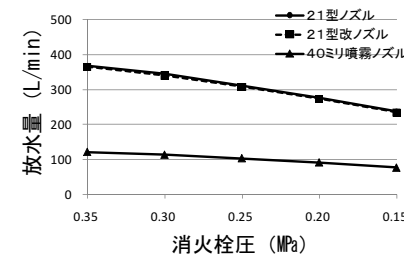
図5 呼称50 3本延長
