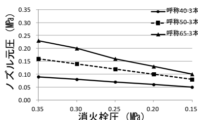
図28 21型ノズル
