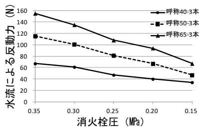
図 35 21型改ノズル
