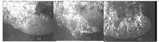
図6 消火器放射中の油面の状況
