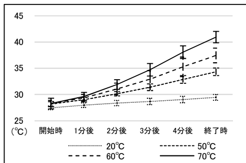
図11 防火衣内温度 (大腿部)
