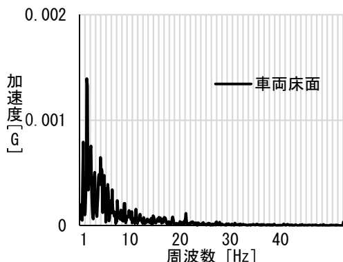
図 3 緊急走行時の救急車両床面の振動に含まれる周波数成分の一例
