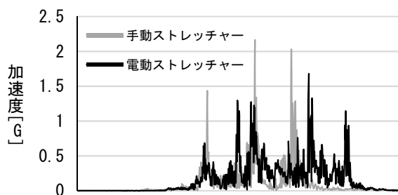
図 12 曳航時における加速度
