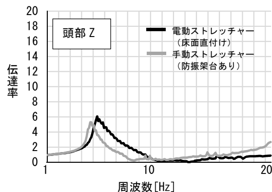
図 5 人体ダミー有の各ストレッチャーの固有振動数を示したグラフの一例
