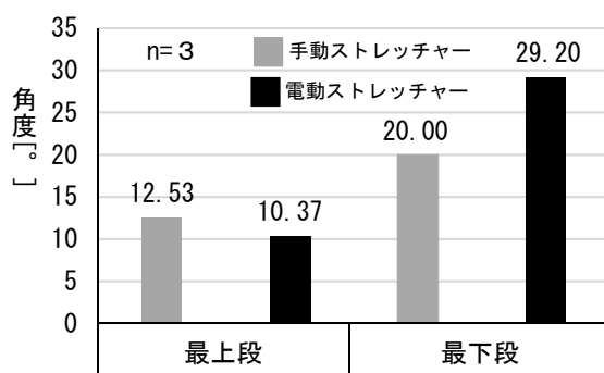
図 11 転倒開始角度の結果
