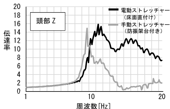
図 4 各ストレッチャーの固有振動数を示したグラフの一例
