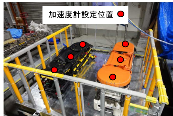
写真8 各ストレッチャー加速度計設定位置
