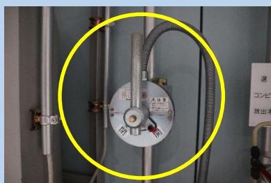
集合管に閉止弁を設置した例
