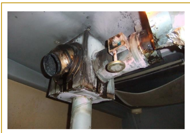
焼損したダクトの外観
